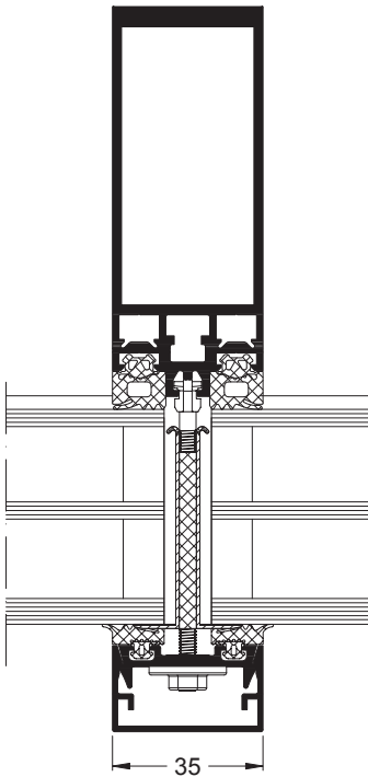
Horizontalschnitt Schüco Fassade FWS 35 PD.SI Maßstab 1:2
