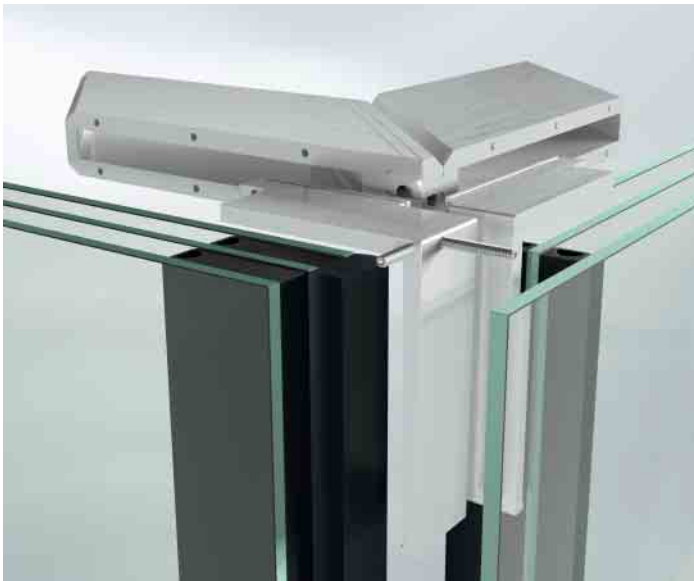
Schüco Fassade FWS 35 PD.SI als Ganzglastecke Schüco Façade FWS 35 PD.SI as all-glass corner
