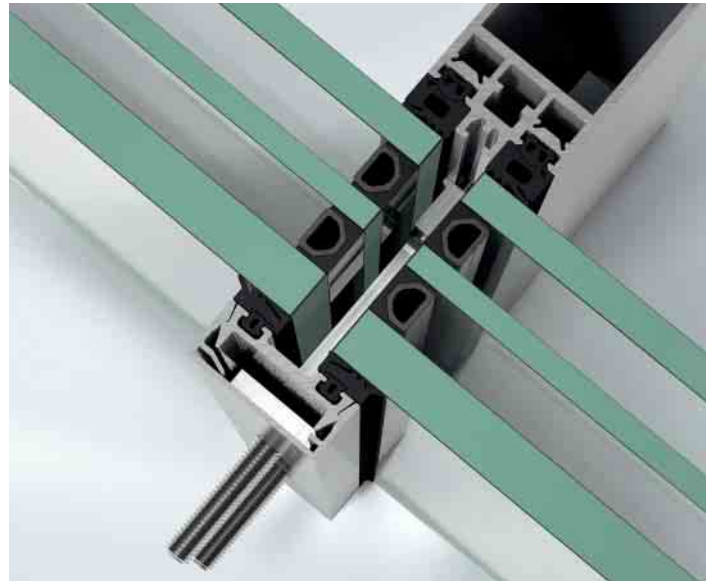
Schüco Fassade FWS 35 PD.SI mit Sonnenschutzbolzen Schüco Façade FWS 35 PD.SI with sun shading bolts
