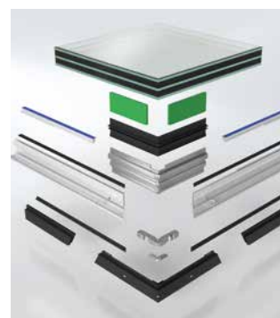
Schüco AWS 75 PD.SI Eckausbildung Schüco AWS 75 PD.SI corner construction
