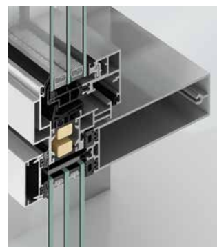
Schüco AWS 75 PD.SI Fassadeneinsatz Schüco AWS 75 PD.SI façade insert
